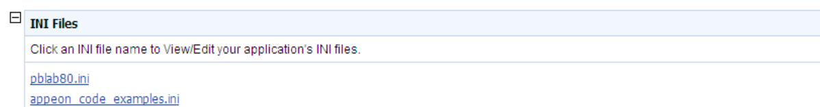
Figure 5.74: INI files
