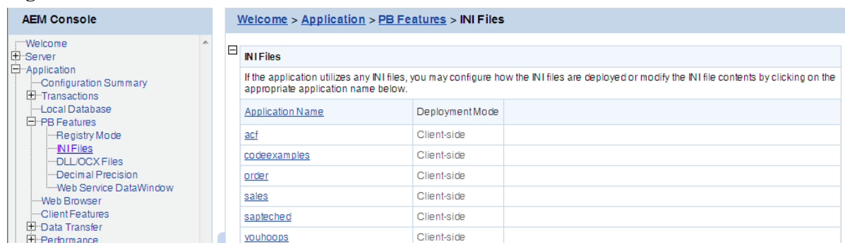
Figure 5.73: INI files
