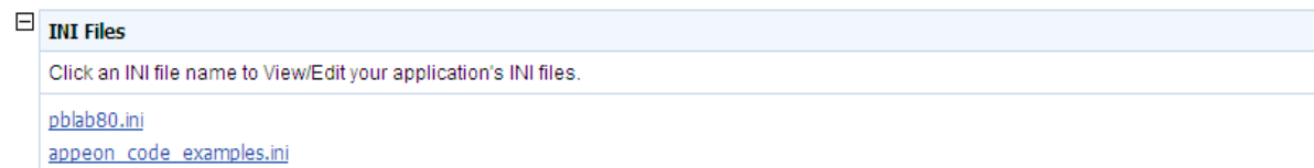
Figure 5.75: INI files
