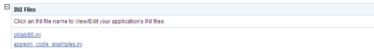
Figure 5.68: INI files
