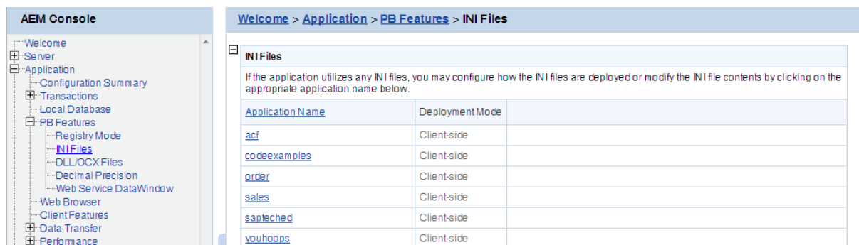
Figure 5.66: INI files
