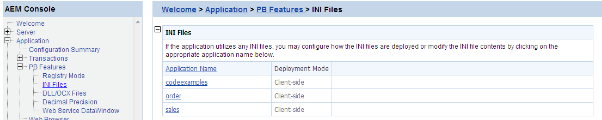
Figure 5.64: INI files
