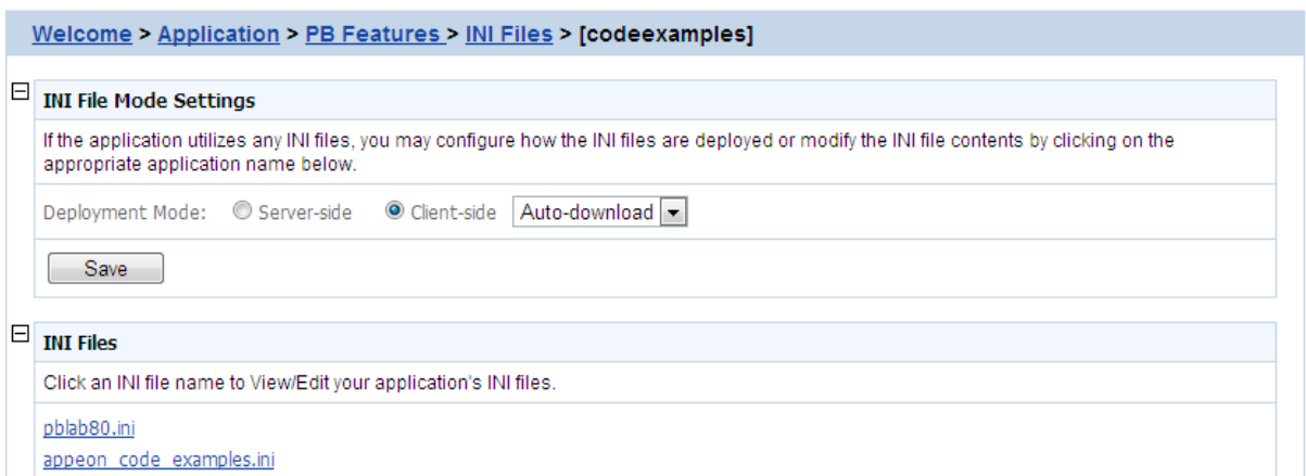
Figure 5.65: INI file mode settings
