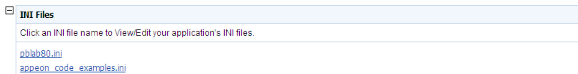
Figure 5.66: INI files
